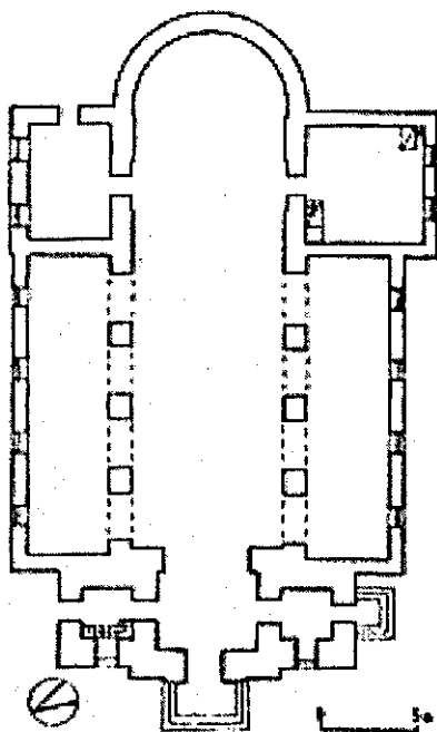
Lyduokių bažnyčios planas
