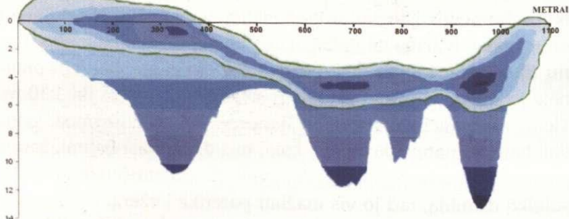
ŽEMAITKIEMIO EŽERO DUGNO PROFILIS
