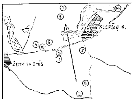
Žemaitkiemio meteorito kritimo schema: skaičiai žymi rastų meteoritų vietas; rodyklė – meteoritų kritimo kryptį
